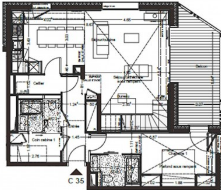
PLAN - NIVEAU 3 (Accès)
