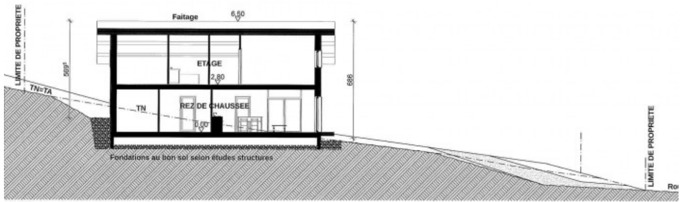
PCMI 03 : COUPE SUR TERRAIN ET CONSTRUCTION
